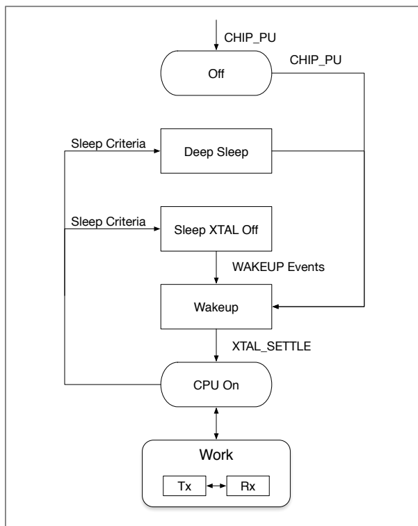
图 3-2. 低功耗管理
